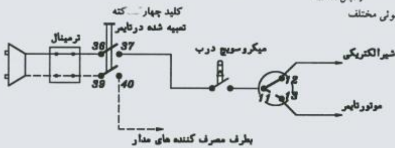
تسمتی از مدار سیم‌بندی ماشین آزمایش مدل ۲۰۰۱
