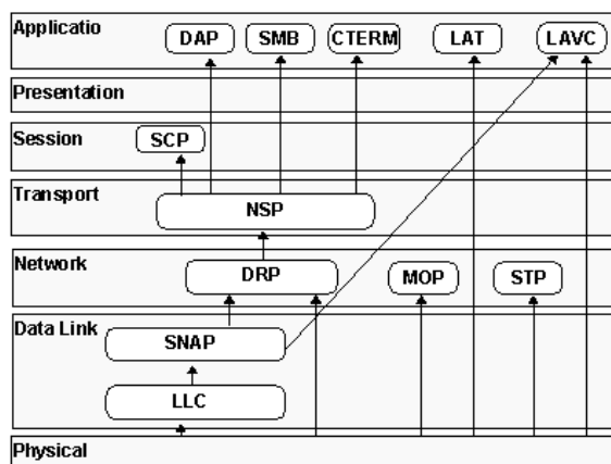
نمایش مجموعه پروتکل DECnet بر اساس لایه بندی مدل OSI
